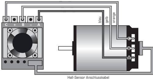
Hall-Sensor Anschlusskabel
